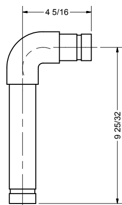
ELEVATION SCALE: 1/3
