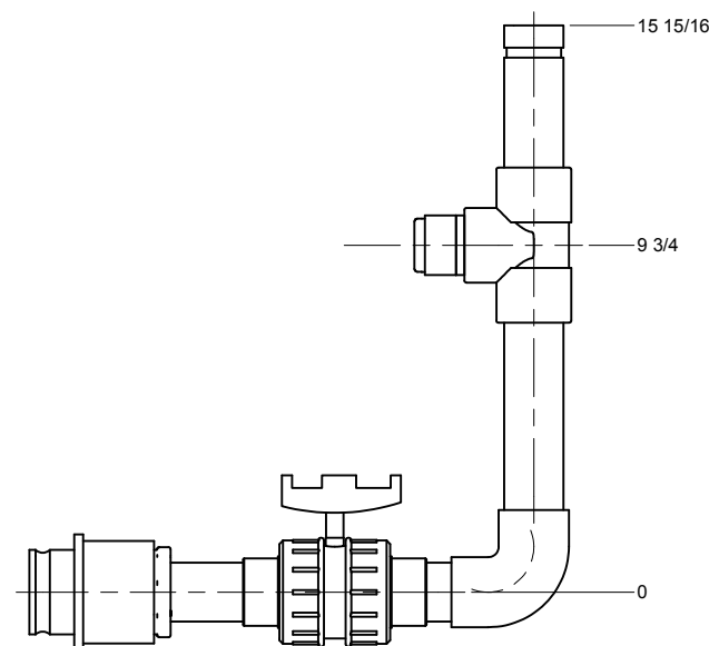
ELEVATION SCALE: 1/3
