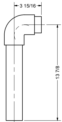
ELEVATION SCALE: 1/4
