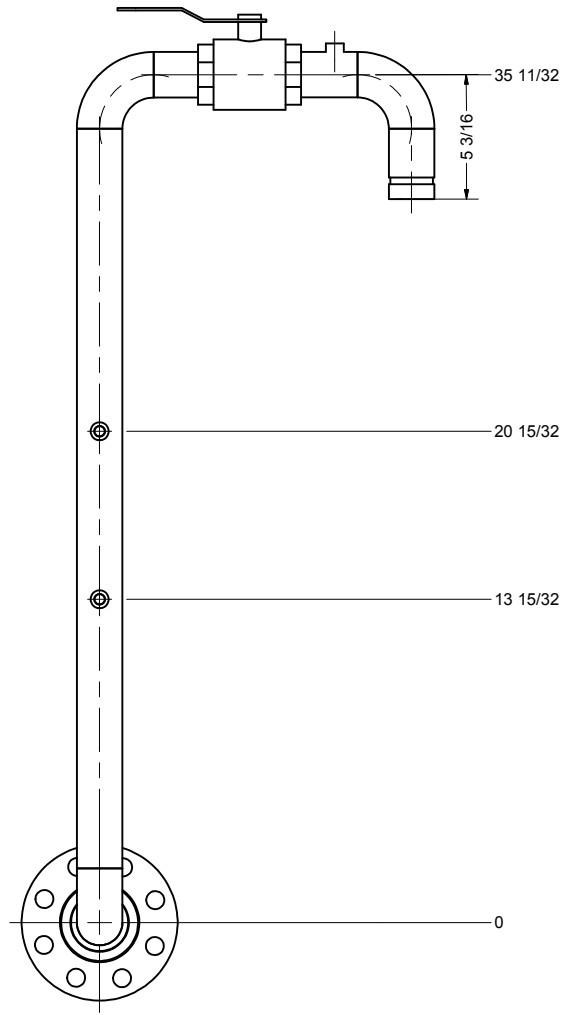
ELEVATION SCALE: 1/4
